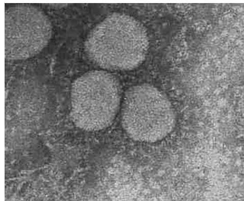
SARS Coronavirus
