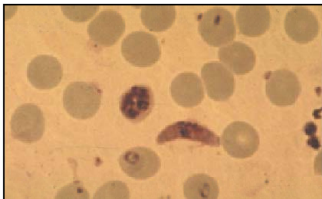
Plasmodium Falciparum
